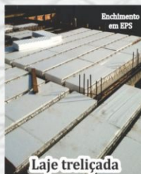
Laje treliçada
